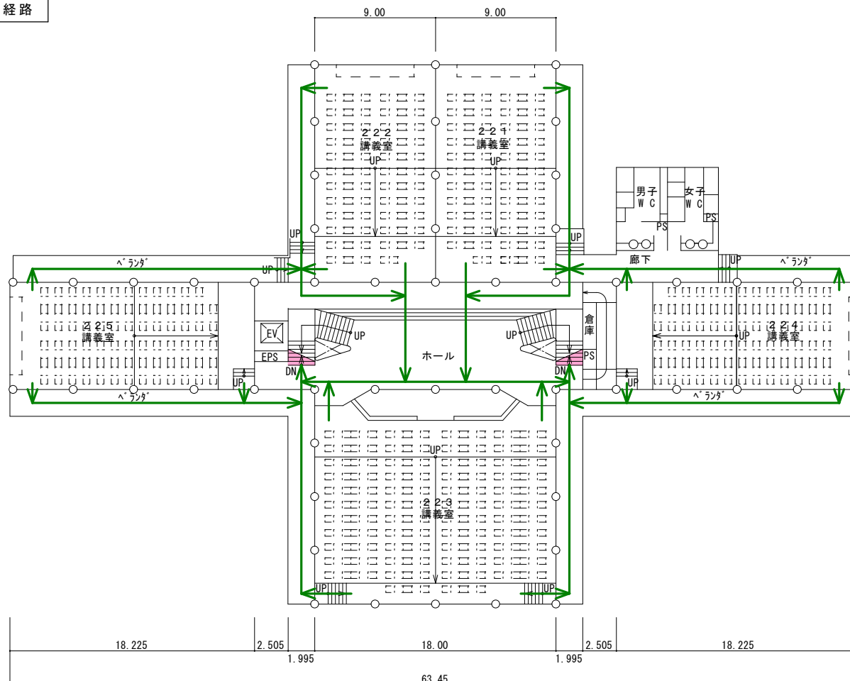
2階平面図
