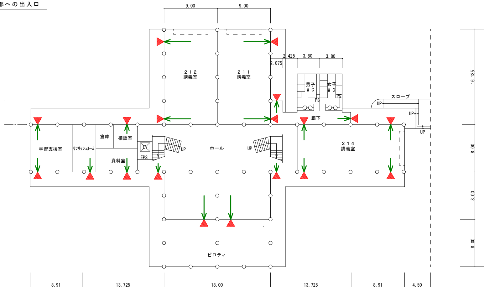
1階平面図
