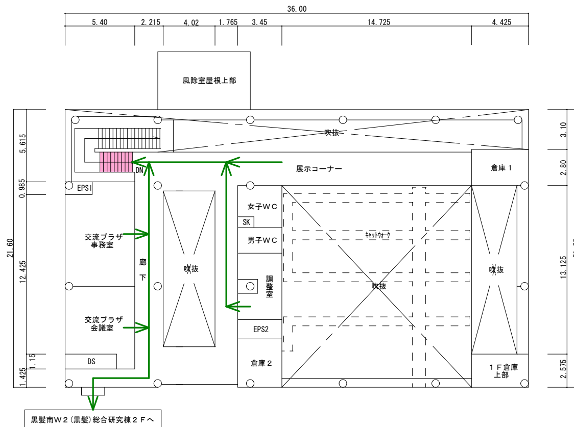
2階平面図
