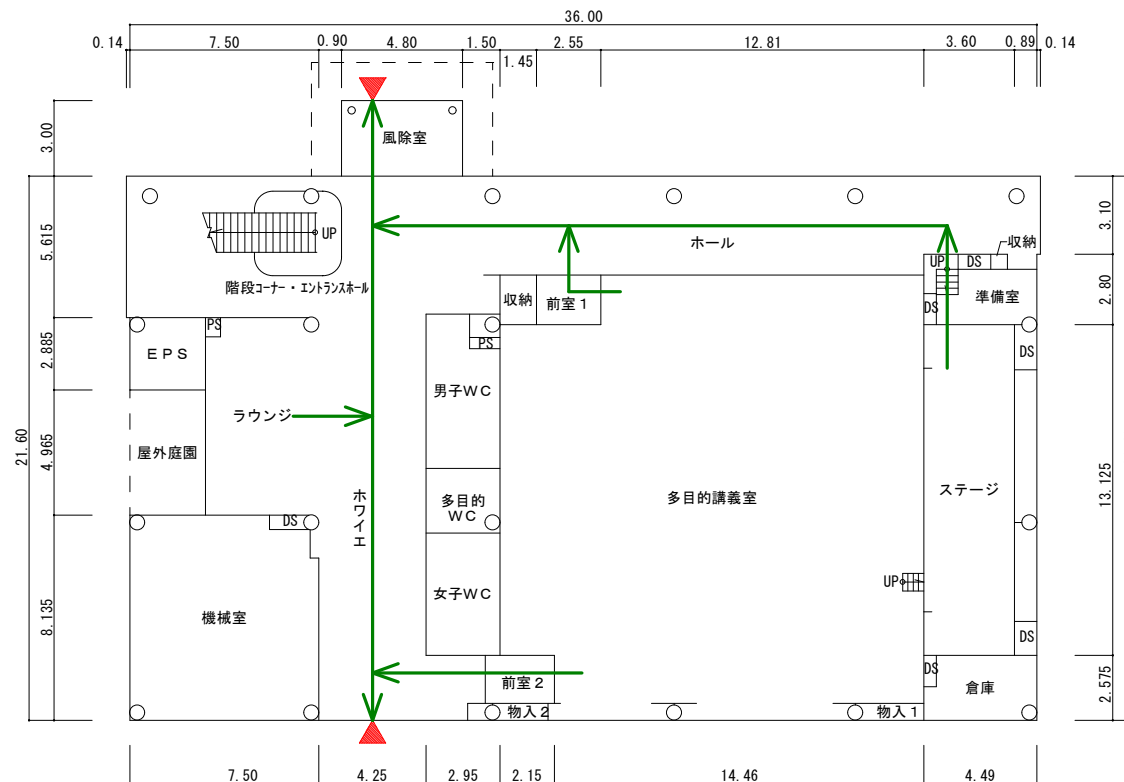
1階平面図
