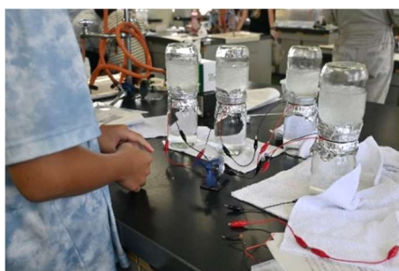
写真5 お湯と氷水による発電実験
