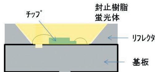
図3 LEDの構造
