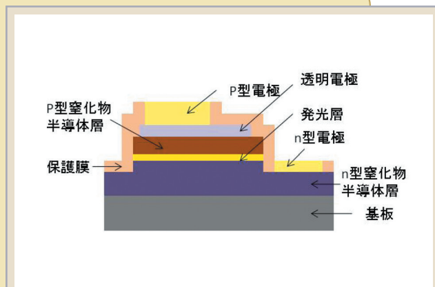
図4 チップ断面構造
